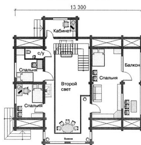
ПЛАН МАНСАРДЫ
