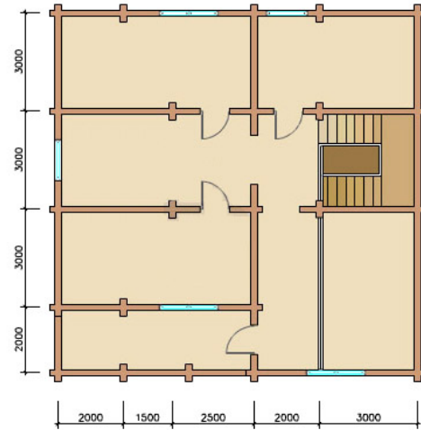
ПЛАН МАНСАРДЫ
