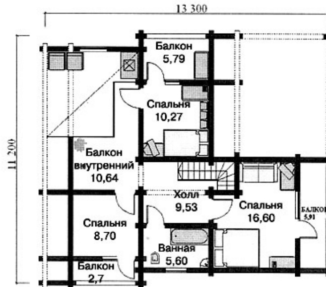
План 2 этажа
