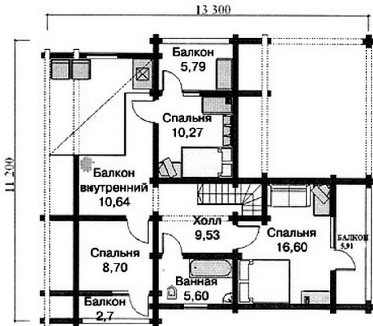
План 2 этажа
