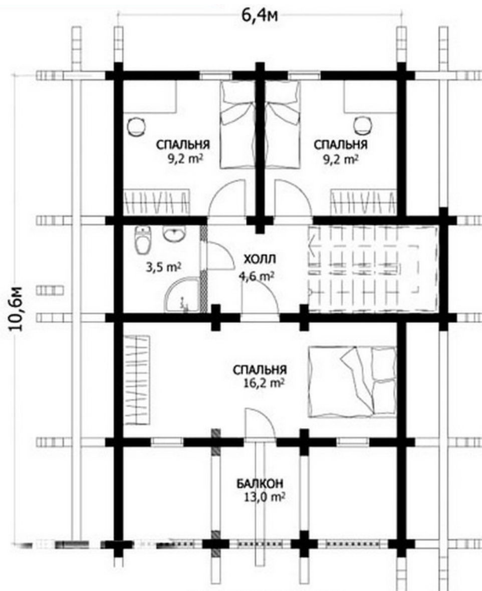
ПЛАН МАНСАРДЫ
