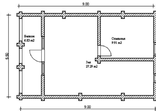
План мансарды
