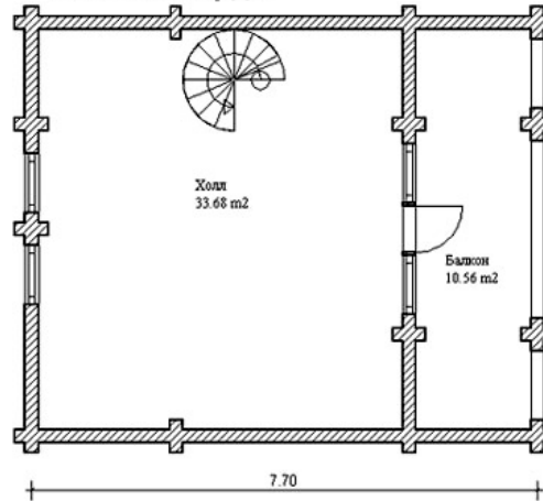
План мансарды
